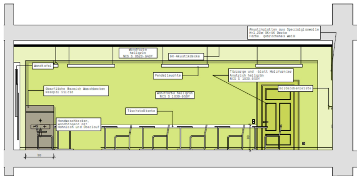
MUSTERKlassenraum BIOLOGIE - Altbau / 1:50 / 03.09.15
