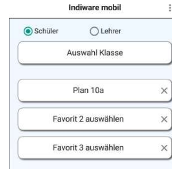
Vertretungsplanapp
